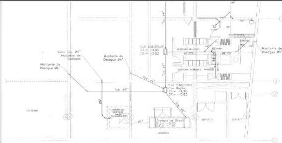
LEVANTAMIENTO PLANTA SEGUNDO SOTANO RED DE DESAGUE DE COCINAS ESC. 1/50
