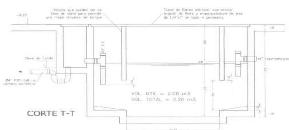
DETALLE DE TRAMPA DE GRASA EXISTENTE
