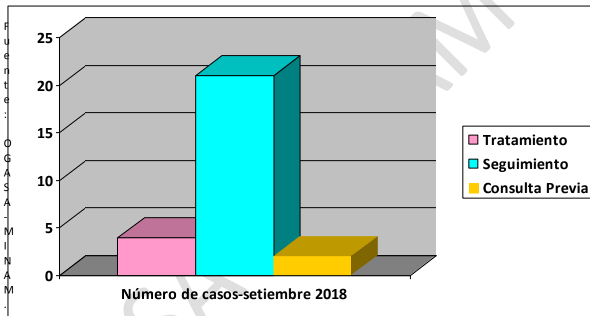
Gráfico n° 1. Número de casos de conflictos socioambientales con participación del MINAM
